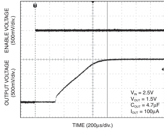
Enable Turn-On
